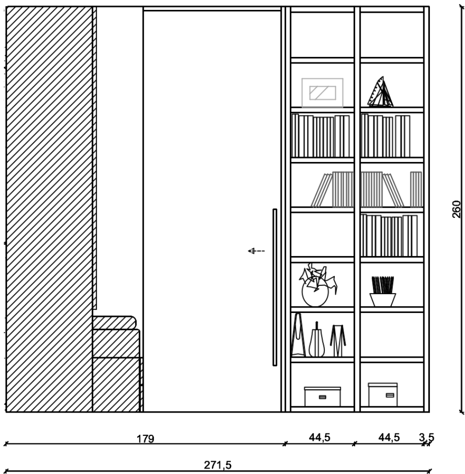
Sezione C
