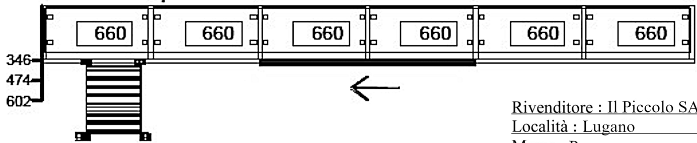
Fronte Aperto - Parete 1
