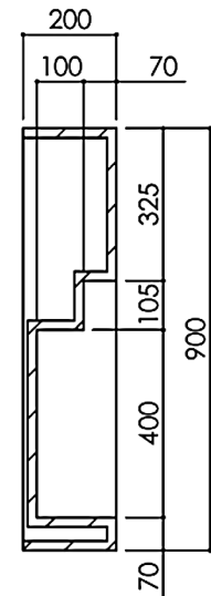
SEZIONE C-C
